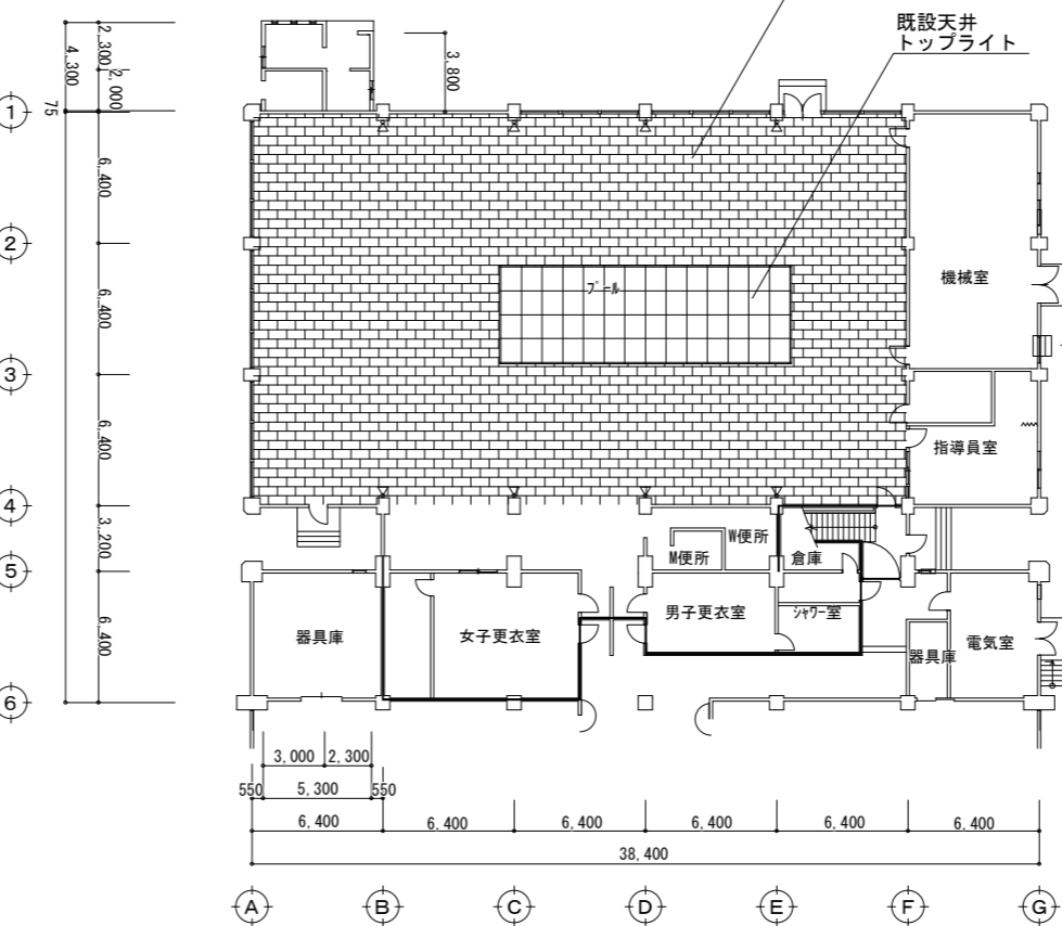
2階天井伏図 1 : 400
