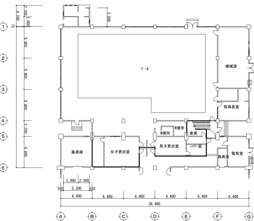
1階平面図 1 : 400
