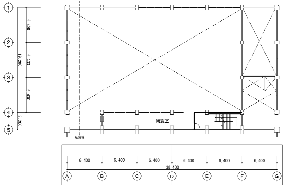
1階天井伏図 1 : 400
