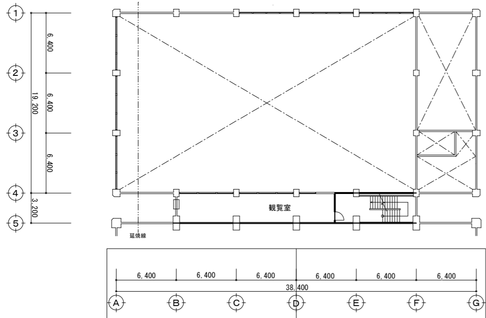
2階平面図 1 : 400
