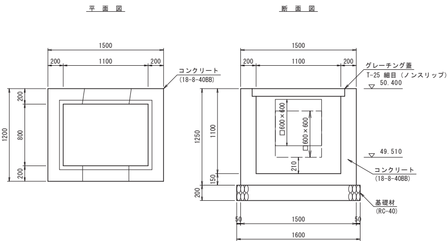
現場打集水樹A S=1:25
