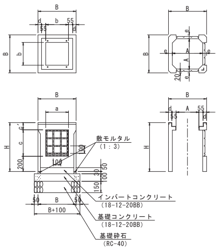
自由勾配側溝用樹 S=1:25
