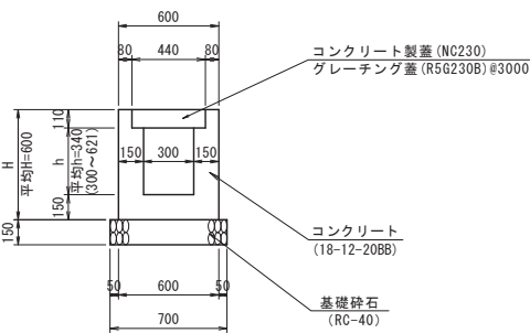
現場打側溝 S=1:25
