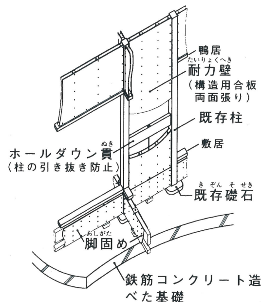
耐力壁と脚固めによる補強
