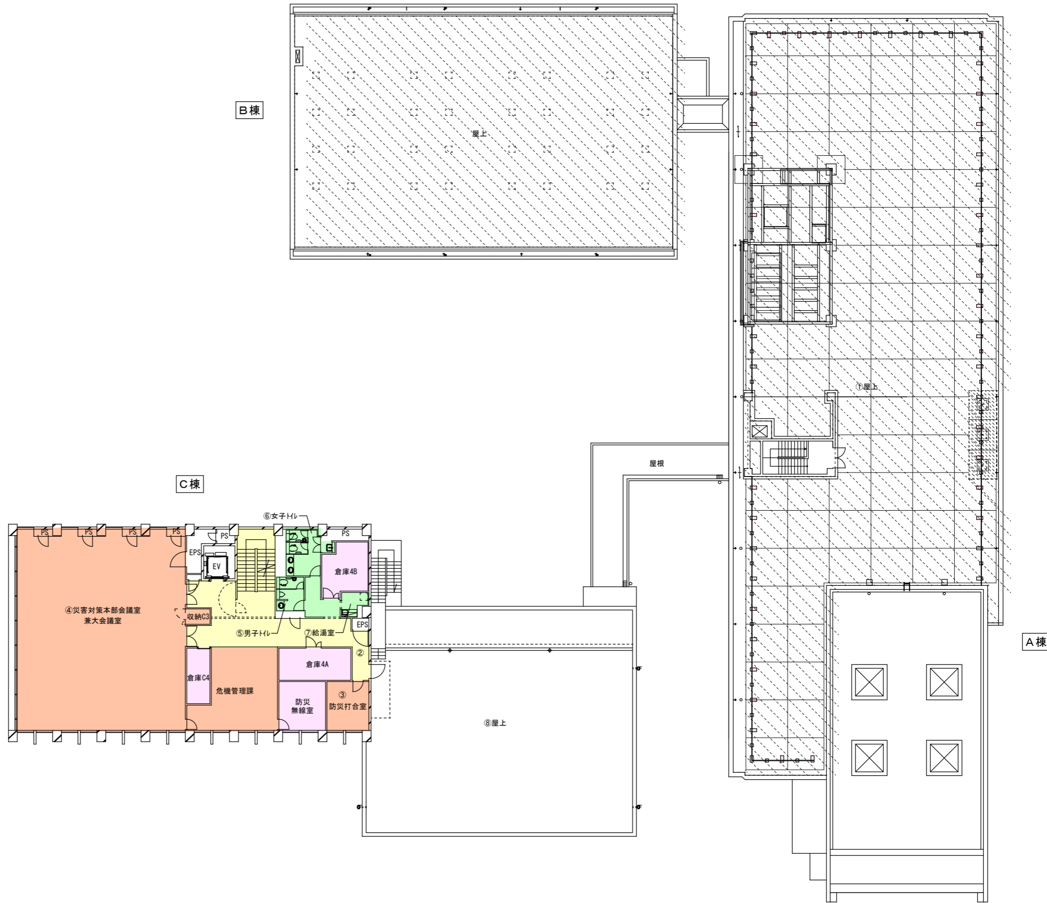
【4階平面図】
