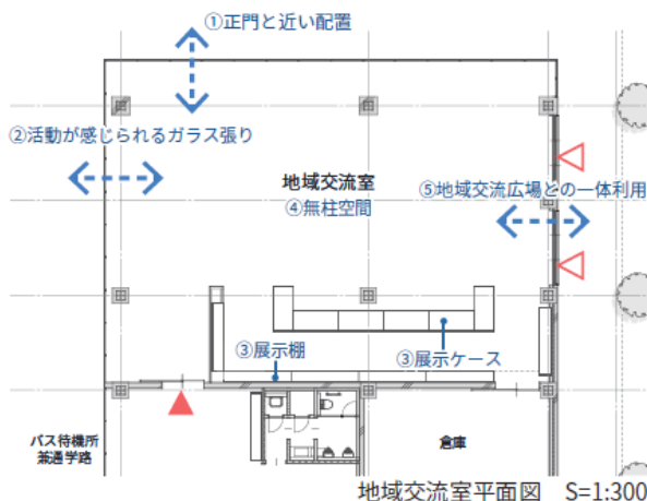
地域交流室平面図 S=1:300
