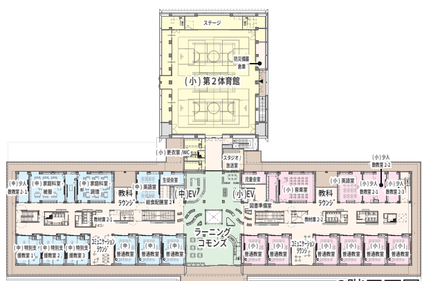
2階平面図
