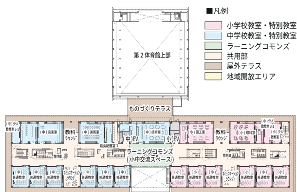
3階平面図
