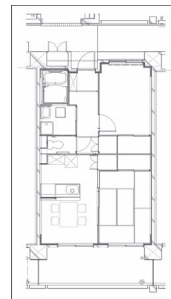
2DK-A 平面図
